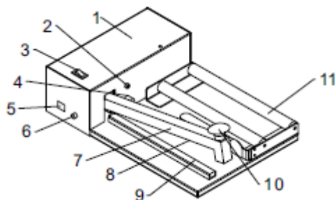
Рис.1 Деталировка:
