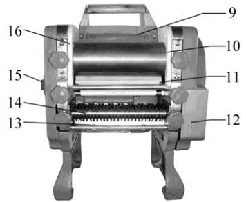
Рис 2: Вид спереди
