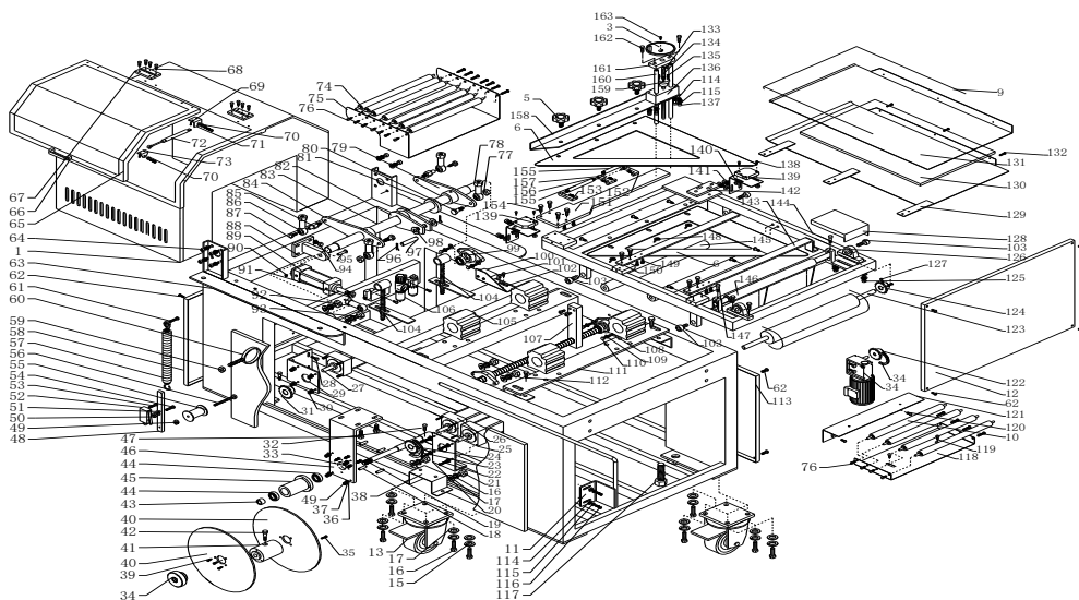
Рис. 2 – Основание машины
