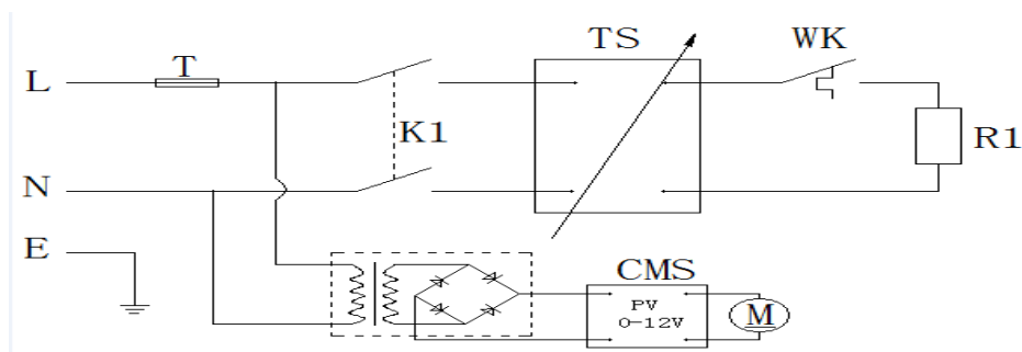
Рис2 – электрическая схема аппарата для приготовления сладкой ваты
