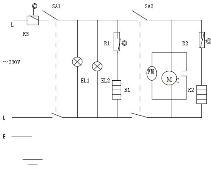
Рис2 – электрическая схема аппарата для приготовления попкорна
