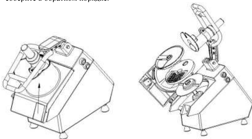
Рис.8 – Смена ножей
