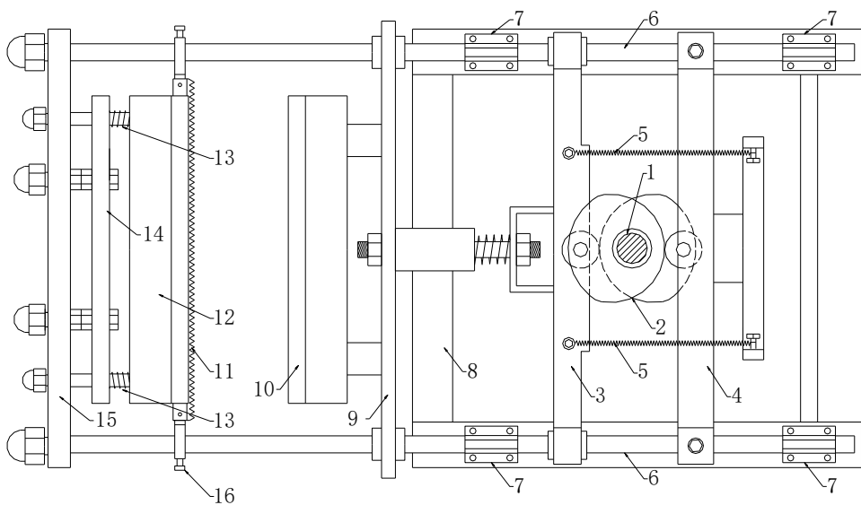
Рис. 5 - Горизонтальный уплотнительный блок
