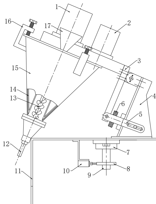
Рис. 3 - Устройство наполнения
