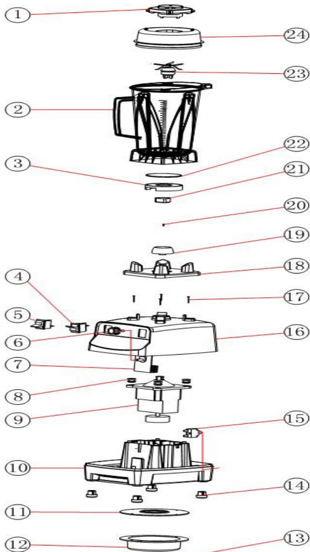
Рис. 1 - Блендер Обозначения
